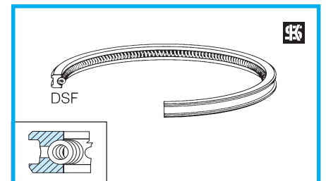
DSF Dachfasen-Schlauchfederring
