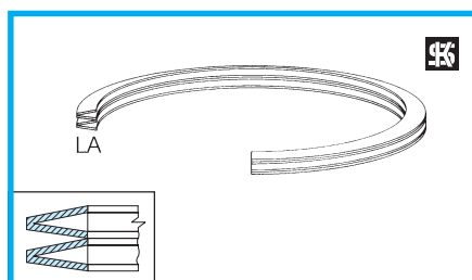
LA Lamellenring
