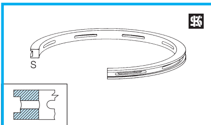
S Ölschlitzring
