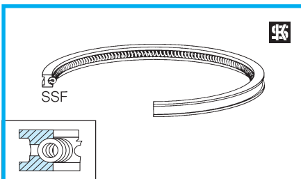
SSF Ölschlitz-Schlauchfederring
