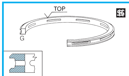
G Gleichfaserring
