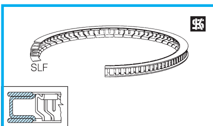
SLF Stahllamellen-Ölring
