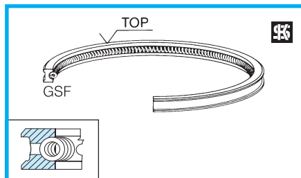
GSF Gleichfasen-Schlauchfederring
