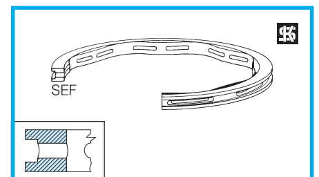
SEF Ölschlitzring mit Expanderfeder
