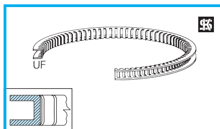
UF U-Flex-Ring
